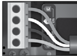
230 V (4 fils - biphasé)
